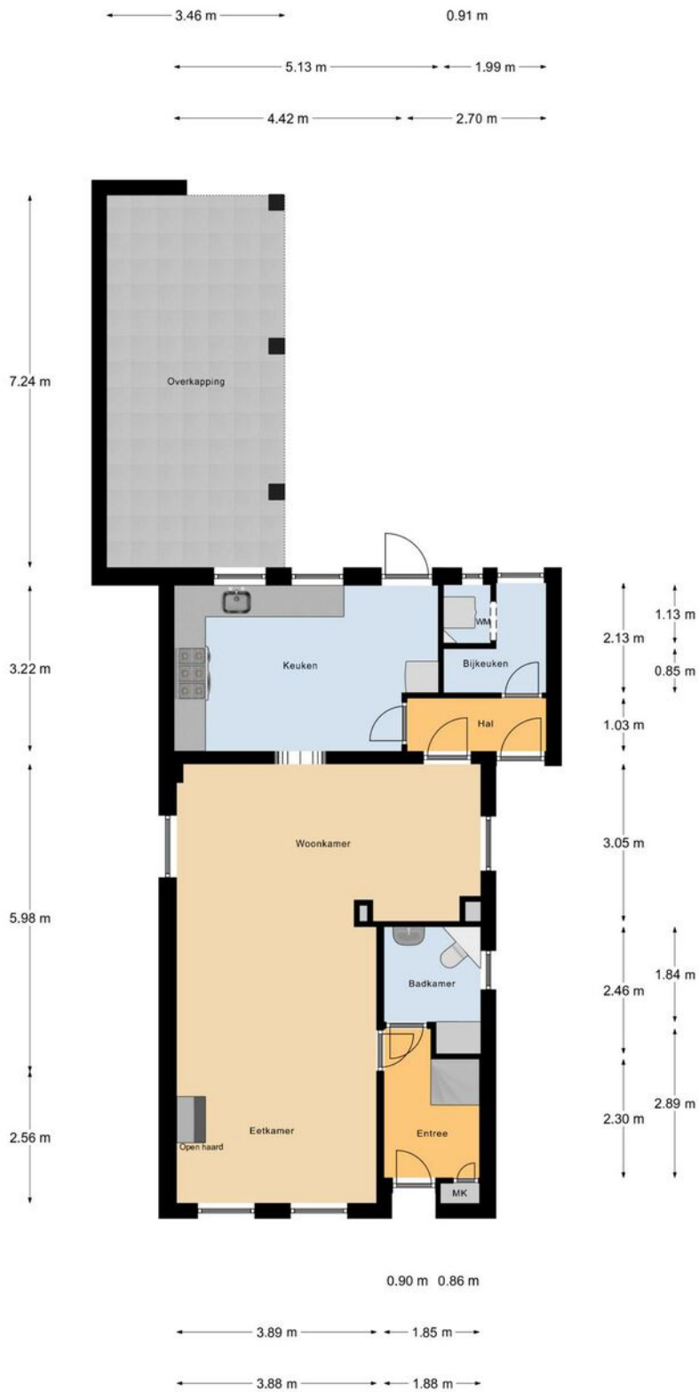
Begane Grond
